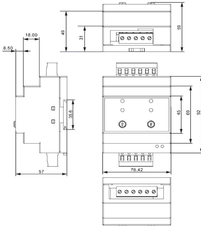
Figura 5 - Dimensões do controlador
