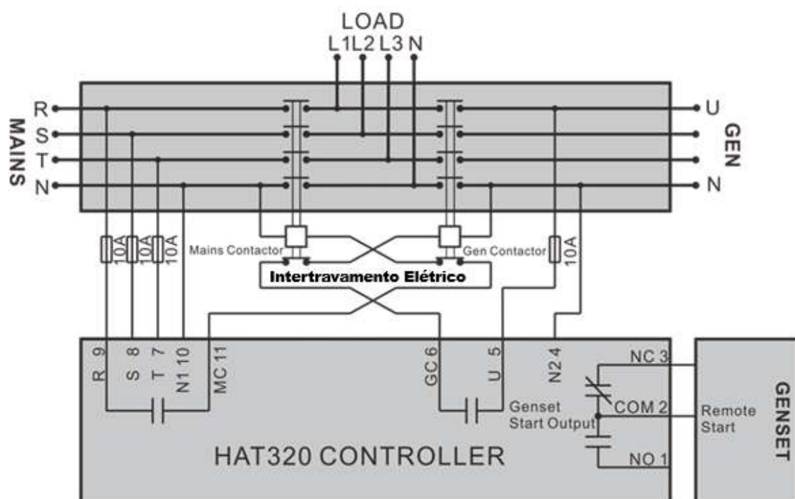
Figura 3 - Diagrama Série HAT320 com Contadores
