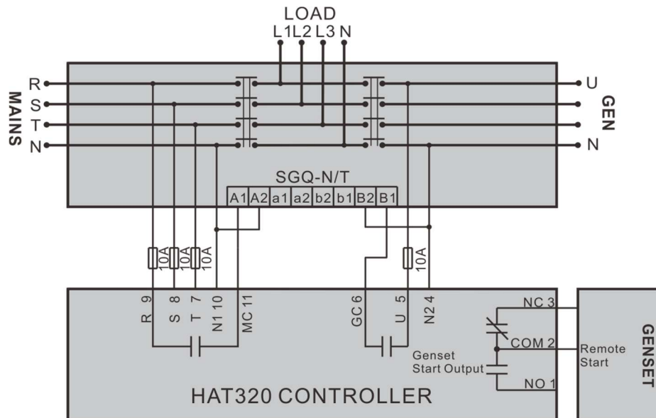
Figura 4 - Diagrama Série HAT320 com chave SGQ-N/T
