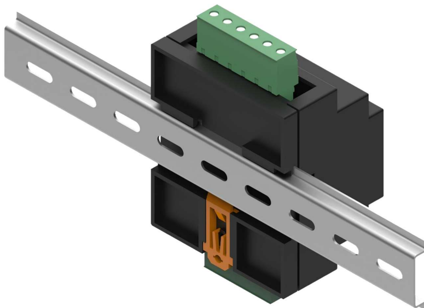
Figura 6 – Instalação via trilho-din 35mm
